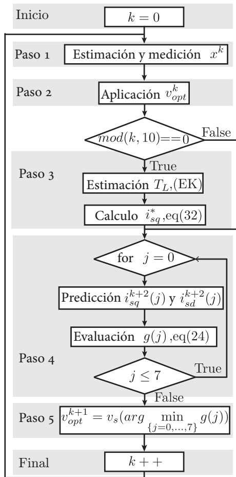
Fig. 3.3. Diagrama de flujo del sistema de control.
