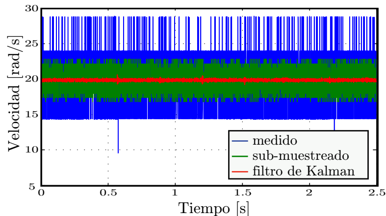
Fig. 6.9. Comparación de velocidad medida, sub-muestreada y estimada mediante el filtro de Kalman.
