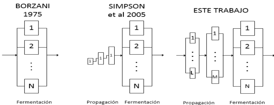
FIGURA 1 RESUMEN DE MÉTODOS DE DISEÑO DE FERMENTACIÓN DISCONTINUA
