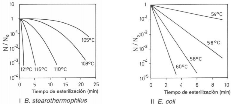
FIGURA 3 CURVAS DE ESTERILIZACIÓN DE B. STEROTHERMOPHILUS Y E. COLI A DISTINTAS TEMPERATURAS.
