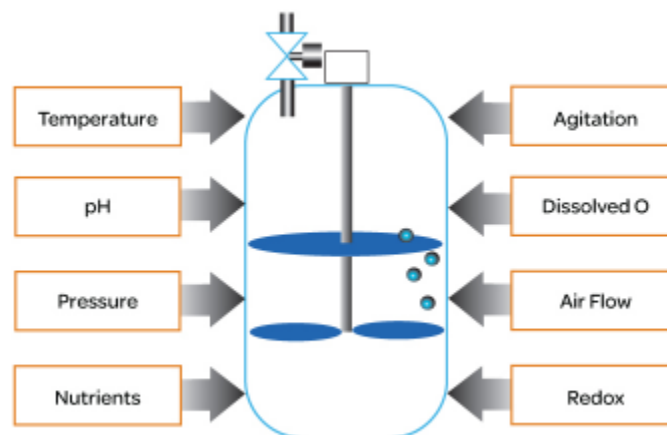
FIGURA 5 VARIABLES DE PROCESO DE FERMENTACIÓN.
