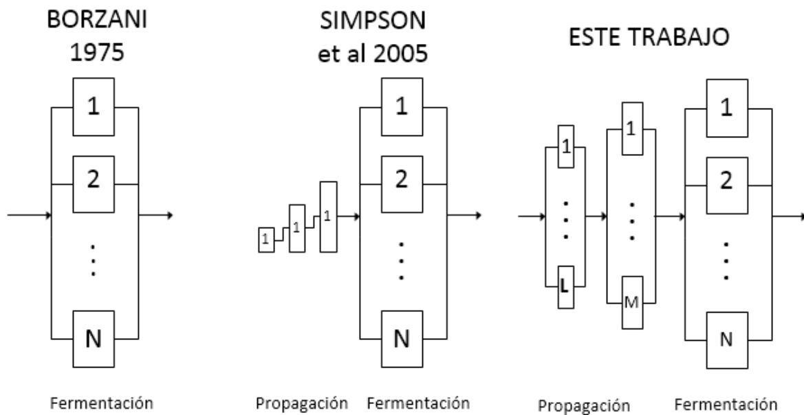
FIGURA 19 COMPARACIÓN DE MÉTODOS DE DISEÑO DE PLANTAS LOTE
