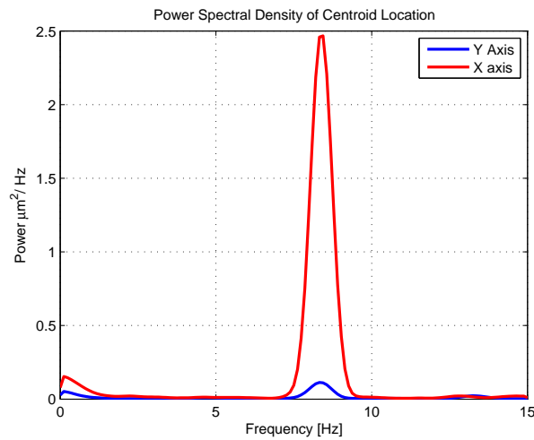
Figura 4.2: Densidad espectral de potencia de la posición del sin control en ambos ejes
