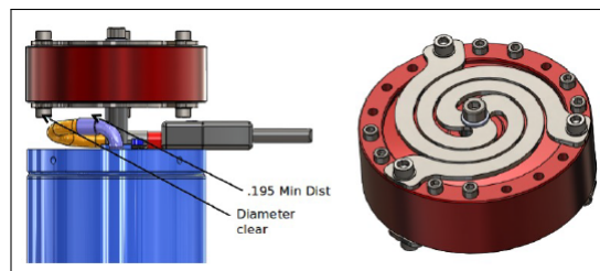
Figura 1.2: TVA montado sobre un enfriador criogenico del GPI
