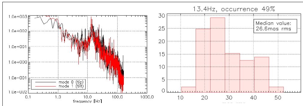
Figura 2.15: Vibraciones sobre el espejo secundario
