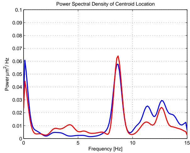
Figura 4.3: Densidad Espectral de Potencia del movimiento del centroide con control en ambos ejes
