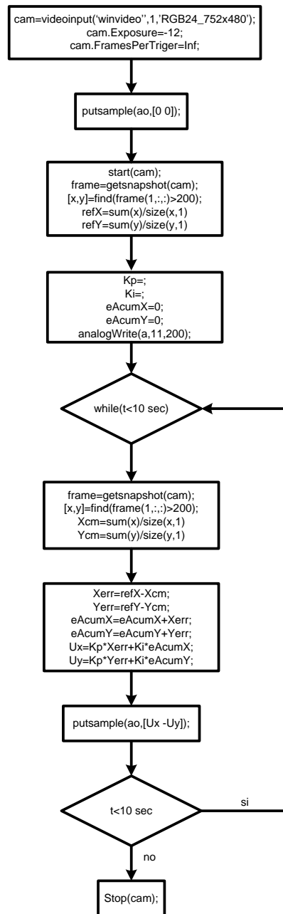
Figura 4.1: Lazo de control programado en matlab
