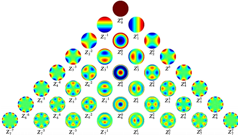
Figura 2.5: Ilustración piramidal de Polinomios de Zernikes hasta el séptimo orden. La notación contiene el coeficiente (Z), el orden (subíndice) y la frecuencia radial (superíndice)
