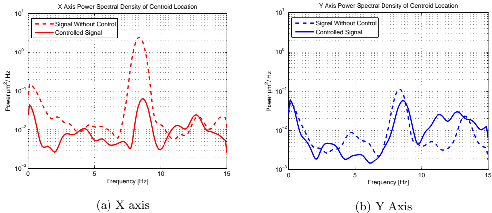
Figura 4.4: Desempeño del lazo de control
