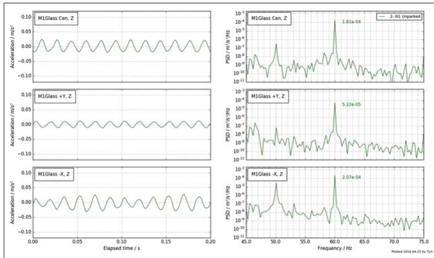
Figura 2.16: Aceleración medida sobre el espejo primario con GPI montado
