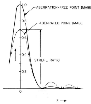
Figura 2.2: Ejemplo de Strehl Ratio S = 0.7
