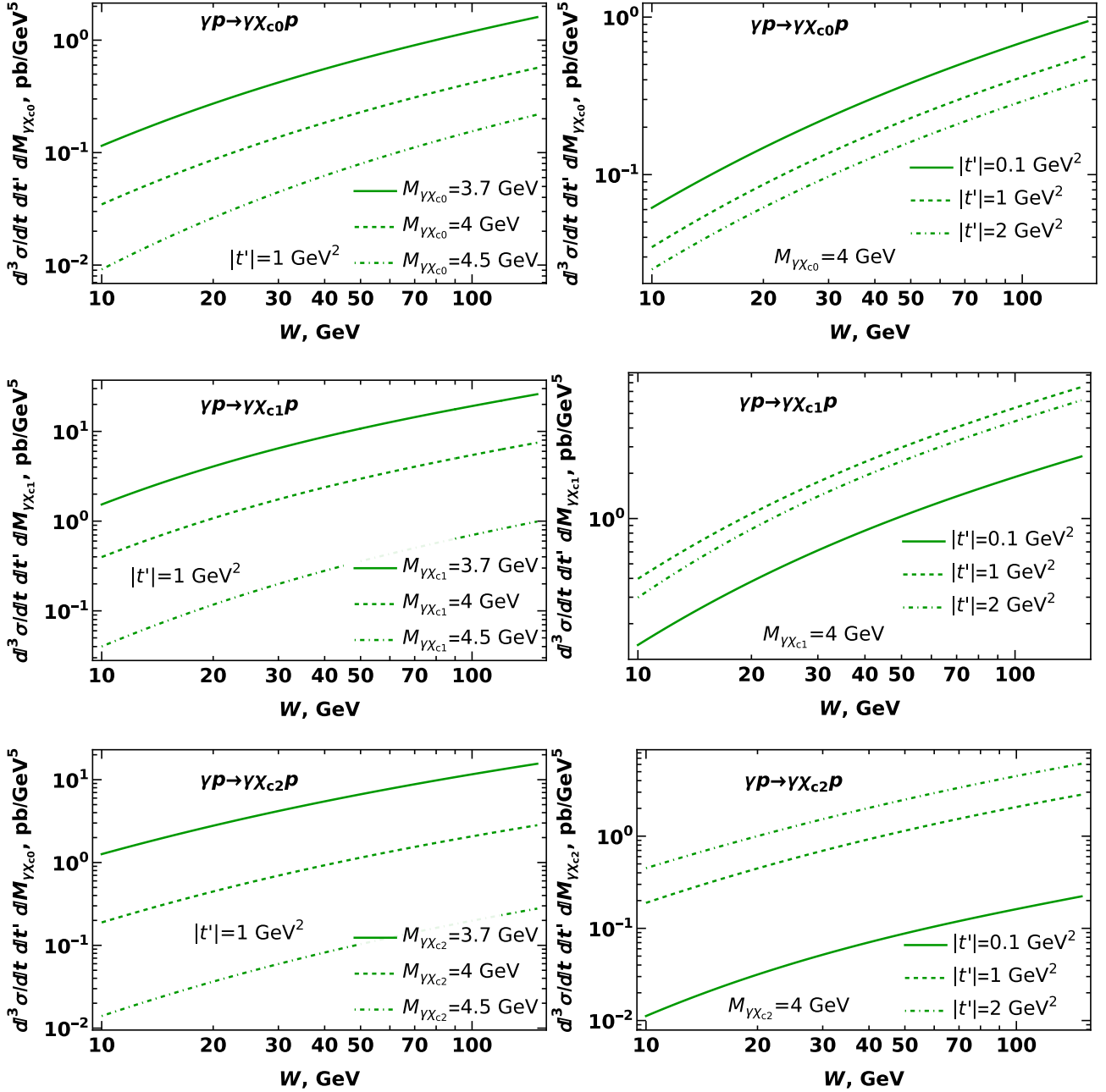
Figura 19: Dependencia de la sección eficaz diferencial en la energía W para \gamma\chi_{cJ} en la factorización colineal.
