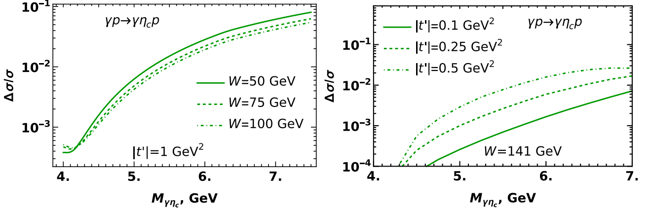
Figura 25: Relación entre las secciones eficaces con y sin cambio de helicidad del fotón como función de la masa invariante del sistema \gamma\eta_c en el marco de la factorización colineal (panel izquierdo) y del CGC (panel derecho).
