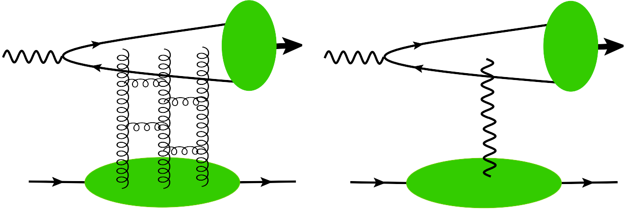
Figura 32: Diagramas esquemáticos de dos mecanismos alternativos de producción exclusiva: a la izquierda, el canal mediado por intercambio de odderón; a la derecha, el mecanismo de Primakoff asociado al intercambio de un fotón.
