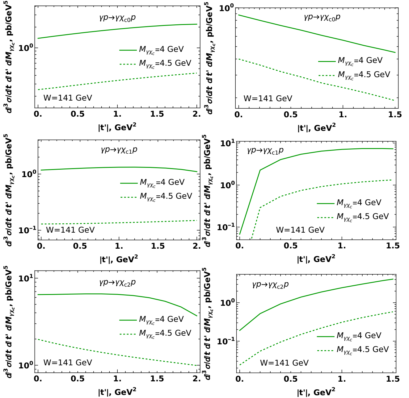
Figura 21: Dependencia de la sección eficaz diferencial en |t'| para \gamma\chi_{cJ} . La columna izquierda corresponde a los resultados obtenidos en el marco del CGC, mientras que la columna derecha muestra los resultados en la factorización colineal.
