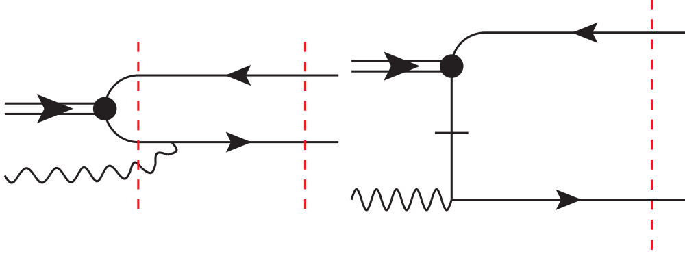
Figura 15: Contribuciones a la función de onda \Psi_{\gamma Q \rightarrow \bar{c}c} asociadas a la emisión del fotón final desde la línea del cuark. A la izquierda se muestra la contribución ordinaria, con un propagador fermiónico intermedio y dos denominadores de energía del cono de luz. A la derecha se muestra la contribución instantánea del propagador, con un único denominador de energía.
