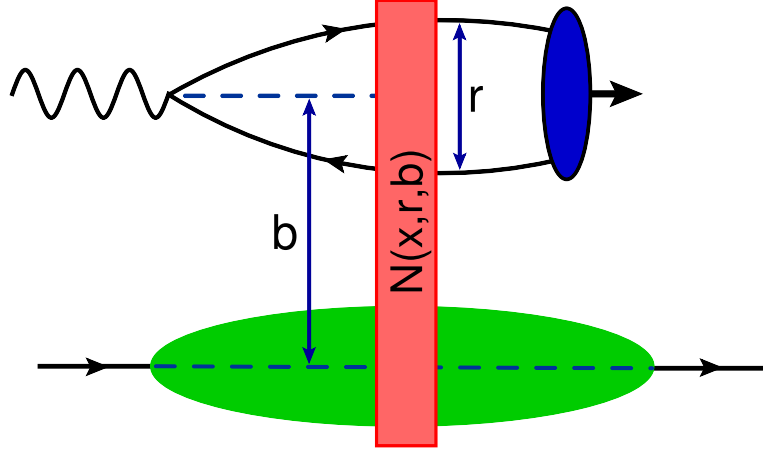
Figura 5: Variables geométricas que parametrizan la amplitud dipolar en el espacio transversal: el tamaño del dipolo \mathbf{r} y su parámetro de impacto \mathbf{b} .
