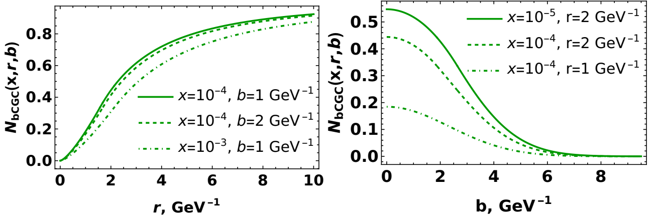
Figura 7: Dependencias de la amplitud dipolar en la parametrización bCGC. Panel izquierdo: N_{\text{bCGC}}(x, \mathbf{r}, \mathbf{b}) como función del tamaño dipolar \mathbf{r} , mostrando la transición desde transparencia de color ( N \ll 1 cuando \mathbf{r} \rightarrow 0 ) hacia el límite de disco negro ( N \rightarrow 1 para valores grandes de \mathbf{r} ). Panel derecho: N_{\text{bCGC}}(x, \mathbf{r}, \mathbf{b}) como función del parámetro de impacto \mathbf{b} , reflejando el decaimiento exponencial del perfil transversal del blanco.
