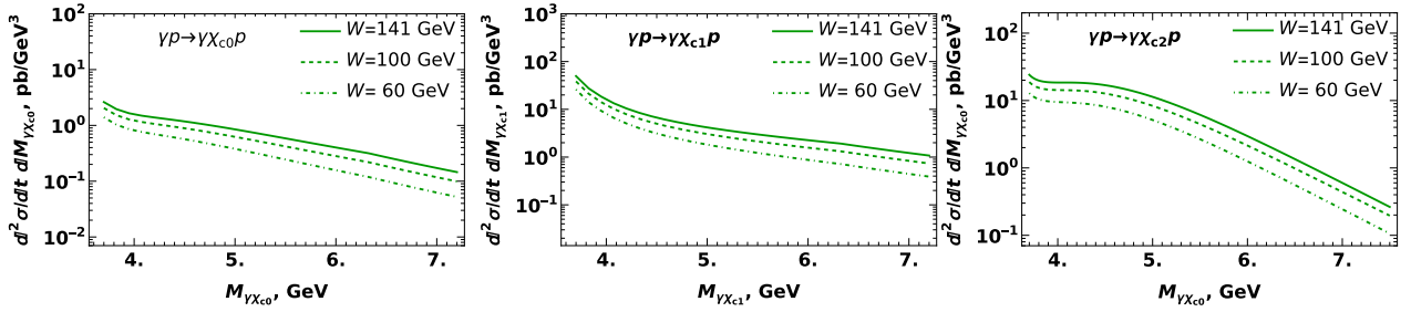
Figura 23: Dependencia de la sección eficaz diferencial en la masa invariante M_{\gamma\chi_{cJ}} en el marco de la factorización colineal.
