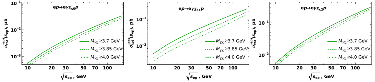
Figura 31: Predicciones en el marco de la factorización colineal para la sección eficaz total de la electroproducción de \gamma\chi_{cJ} en función de la energía \sqrt{s_{ep}} , para distintos cortes en la masa invariante de los pares \gamma\chi_{cJ} .
