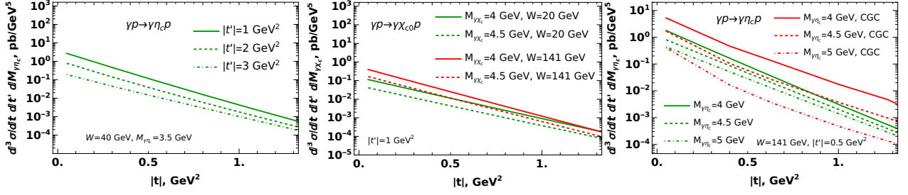
Figura 17: Dependencia en |t| de la sección eficaz diferencial. Panel izquierdo: resultados para distintos valores de |t'| en el marco de la factorización colineal. Panel central: comparación de los resultados para W = 20 y W = 141 GeV en el marco de la factorización colineal. Panel derecho: comparación entre los resultados obtenidos en la factorización colineal (líneas verdes) y en el marco del CGC (líneas rojas).
