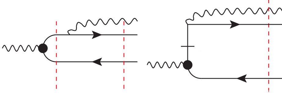
Figura 14: Contribuciones a la función de onda \Psi_{\gamma \rightarrow \gamma \bar{c}c} asociadas a la emisión del fotón final desde la línea del cuark. A la izquierda se muestra la contribución ordinaria, con un propagador fermiónico intermedio y dos denominadores de energía del cono de luz. A la derecha se muestra la contribución instantánea del propagador, con un único denominador de energía. La línea fermiónica vertical con una pequeña barra horizontal denota la parte instantánea del propagador del cuark. Las líneas verticales rojas indican los estados intermedios que generan los correspondientes denominadores de energía.
