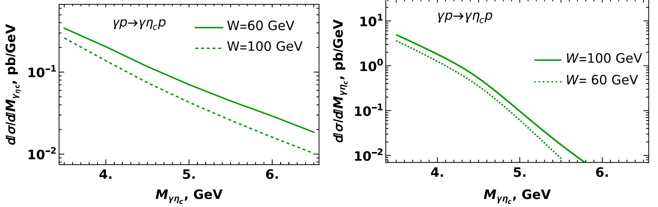
Figura 22: Dependencia de la sección eficaz diferencial en la masa invariante M_{\gamma\eta_c} en el marco de la factorización colineal (panel izquierdo) y del CGC (panel derecho).
