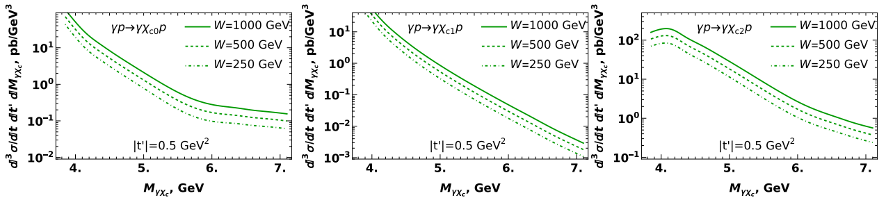
Figura 24: Dependencia de la sección eficaz diferencial en la masa invariante M_{\gamma\chi_{cJ}} en el marco del CGC.
