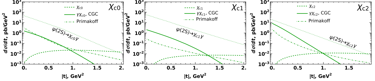
Figura 34: Comparación de la sección eficaz diferencial para distintos mecanismos que contribuyen a la electroproducción exclusiva de \chi_{cJ} y de \gamma\chi_{cJ} (con el fotón final no detectado) a \sqrt{s_{ep}} = 140\text{ GeV} . Las curvas sólidas corresponden al proceso directo ep \rightarrow e\gamma\chi_{cJ}p calculado en el marco del CGC. Las curvas punteadas superiores corresponden a la contribución de pares \gamma\chi_{cJ} procedentes de la desintegración radiativa \psi(2S) \rightarrow \gamma\chi_{cJ} . Las curvas para la electroproducción exclusiva ep \rightarrow e\chi_{cJ}p mediada por odderón y el mecanismo de Primakoff se toman de [55].
