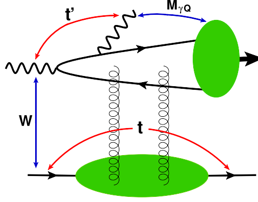
Figura 10: Representación esquemática de la cinemática del proceso exclusivo \gamma p \rightarrow \gamma Q p , con la definición de los invariantes W^2 , t , t' y de la masa invariante M_{\gamma Q}^2 . Las líneas azules conectan los pares de partículas cuyos momentos se suman para formar los invariantes indicados, mientras que las líneas rojas representan diferencias de momentos, tomadas como el momento de la partícula situada a la derecha menos el de la situada a la izquierda.
