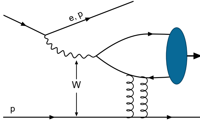
Figura 4: Esquema del proceso exclusivo \gamma p \rightarrow V p a energía W del sistema \gamma p .
