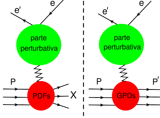
Figura 2: Comparación esquemática entre dispersión ep inclusiva y exclusiva. Izquierda: proceso inclusivo (DIS), en el que el protón se disocia y el estado hadrónico final se trata de forma inclusiva (se indica como X ). Derecha: proceso exclusivo, en el que el protón permanece intacto pero cambia su 4-momento ( P \rightarrow P' ) y se produce un estado final especificado.
