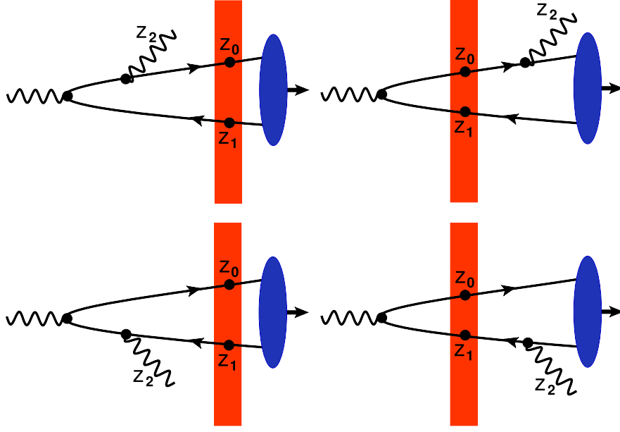
Figura 13: Diagramas que contribuyen a la fotoproducción exclusiva de \gamma\eta_c y \gamma\chi_{cJ} a LO en el marco del CGC. Los diagramas de la izquierda corresponden a la emisión del fotón final antes de la interacción del sistema c\bar{c} con la onda de choque, mientras que los de la derecha describen la emisión después de dicha interacción.
