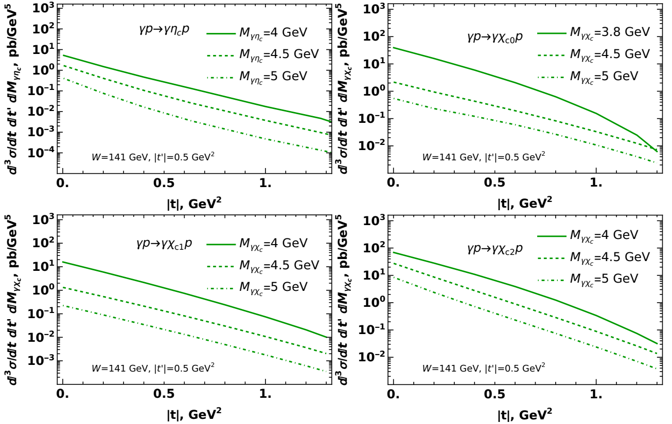
Figura 16: Dependencia de la sección eficaz diferencial en el momento transferido |t| en el marco del CGC.
