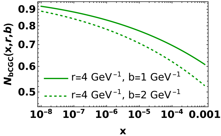
Figura 8: Dependencia en x_{\text{Bj}} de la amplitud dipolar en la parametrización bCGC: N_{\text{bCGC}}(x, \mathbf{r}, \mathbf{b}) como función de x . Al disminuir x , la amplitud crece y muestra una tendencia al aplanamiento, consistente con el régimen de saturación.
