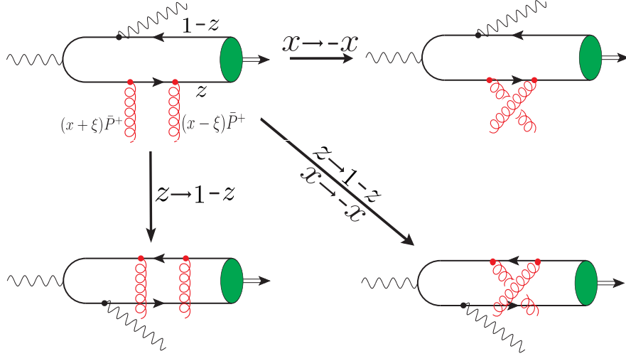
Figura 12: Ilustración, en el ejemplo de un diagrama representativo, de cómo se generan las contribuciones restantes a partir de las simetrías del subproceso. Las operaciones z \rightarrow 1 - z (intercambio cuark-anticuark pesado) y x \rightarrow -x (permutación de las líneas gluónicas en el canal- t ) relacionan los distintos diagramas del conjunto mostrado en la Fig. 11.
