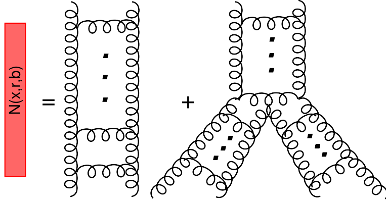
Figura 6: Esquema del contenido físico de la ecuación BK (2.45) para la amplitud dipolar N(x_{Bj}, \mathbf{r}, \mathbf{b}) en el límite de x pequeña: una contribución lineal tipo BFKL (escalera) y una contribución no lineal tipo abanico asociada a la saturación.
