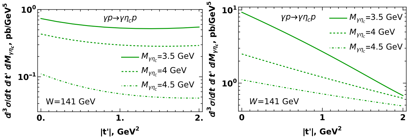
Figura 20: Dependencia de la sección eficaz diferencial en el momento transferido |t'| para \gamma\eta_c en el marco del CGC (panel izquierdo) y de la factorización colineal (panel derecho).
