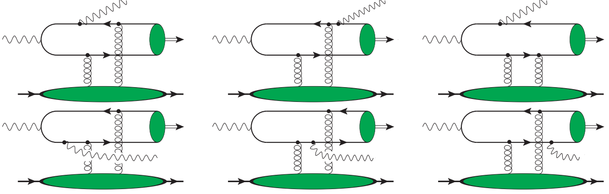
Figura 11: Diagramas de Feynman que contribuyen a la fotoproducción exclusiva del par fotón-mesón a orden líder. A partir de los 6 diagramas representados, los restantes se obtienen mediante el intercambio de las líneas de cuark y anticuark pesados (conjugación de carga) y la permutación de las líneas gluónicas en el canal t . En total, son 24 diagramas que contribuyen. Figura adaptada de la Fig. 4 de [57].
