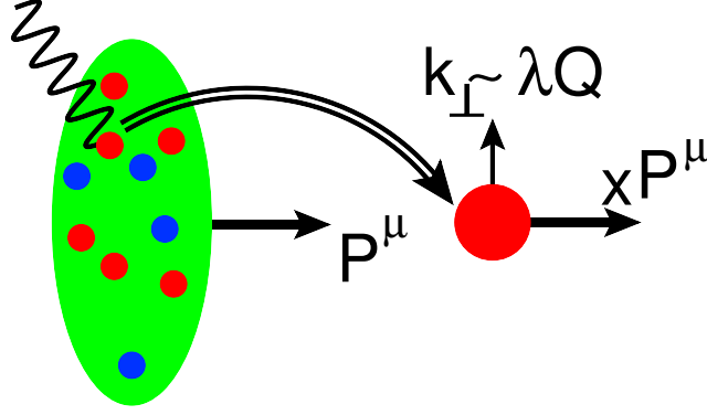
Figura 1: Descomposición del momento del partón activo en coordenadas de cono de luz; la componente paraméricamente pequeña k^- = \mathcal{O}(\Lambda_{\text{QCD}}^2/Q) se omite en el esquema.
