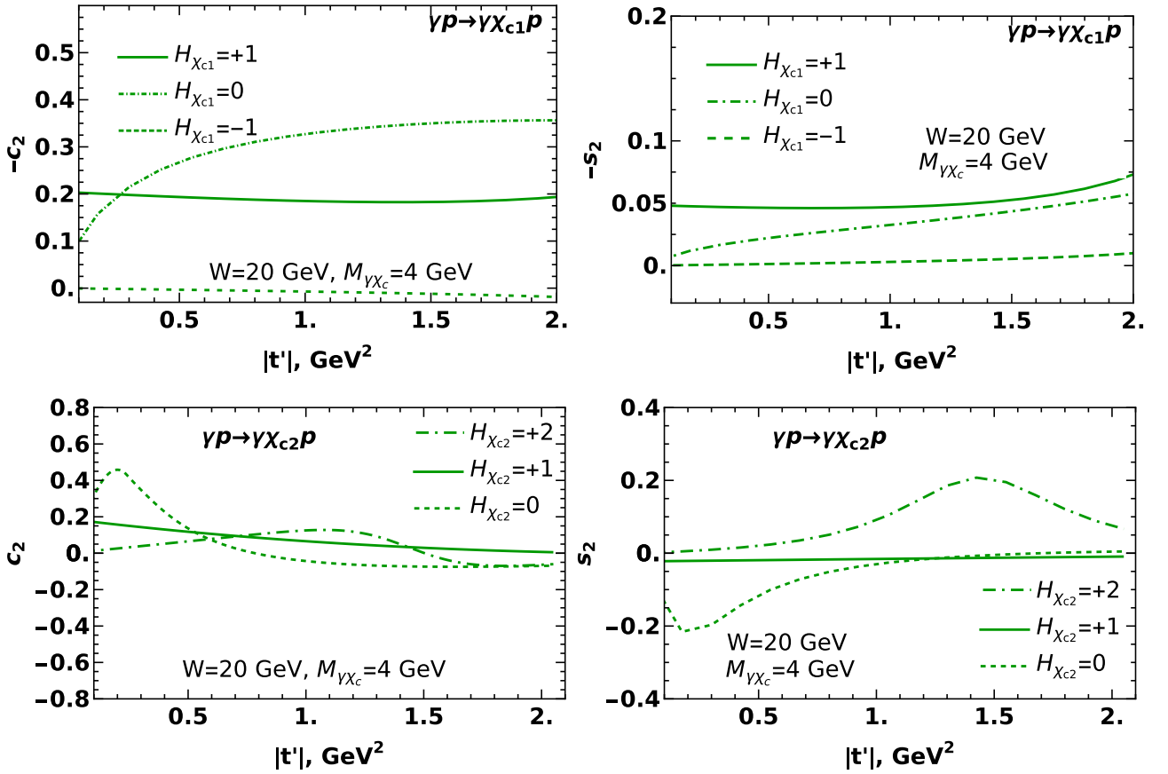
Figura 29: Los armónicos angulares c_2 y s_2 de la sección eficaz de electroproducción (3.24), para distintas componentes de helicidad de los mesones \chi_{c1} y \chi_{c2} en el marco de la factorización colineal (consideramos que la polarización del fotón final es “ -1 ”). No se muestran las asimetrías de las contribuciones con H_{\chi_c} negativas porque son numéricamente despreciables.
