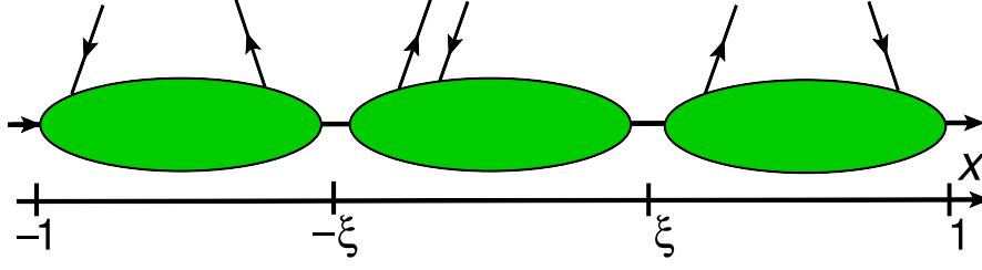
Figura 3: Estructura por regiones de las GPDs en la variable x .
