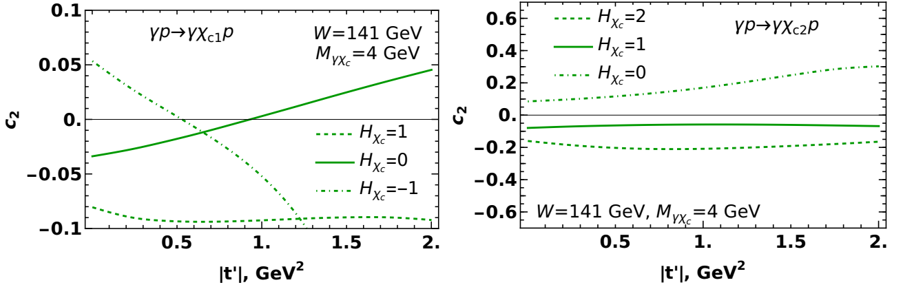
Figura 28: Los armónicos angulares c_2 de la sección eficaz de electroproducción (3.24), para distintas componentes de helicidad de los mesones \chi_{c1} y \chi_{c2} en el marco del CGC (consideramos que la polarización del fotón final es “ -1 ”). En el panel derecho (correspondiente a \chi_{c2} ) no se muestran las asimetrías de las contribuciones con H_{\chi_c} negativas porque son numéricamente despreciables. Además, se supone que el parámetro \epsilon , definido en (3.22), tiene el valor \epsilon = 0,5 .
