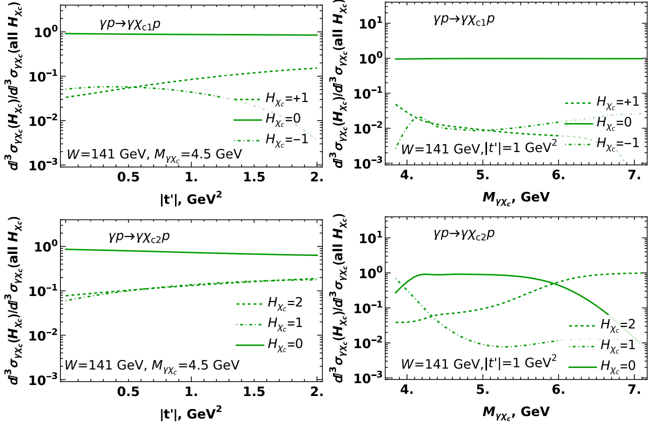
Figura 27: Las contribuciones relativas de las distintas componentes de helicidad de \chi_{c1} y \chi_{c2} a la sección eficaz diferencial, como función de las variables cinemáticas t' y M_{\gamma\chi_c} (en el marco del CGC). En la línea inferior (correspondiente a \chi_{c2} ) no se muestran las contribuciones, numéricamente despreciables, de las componentes con helicidad negativa.
