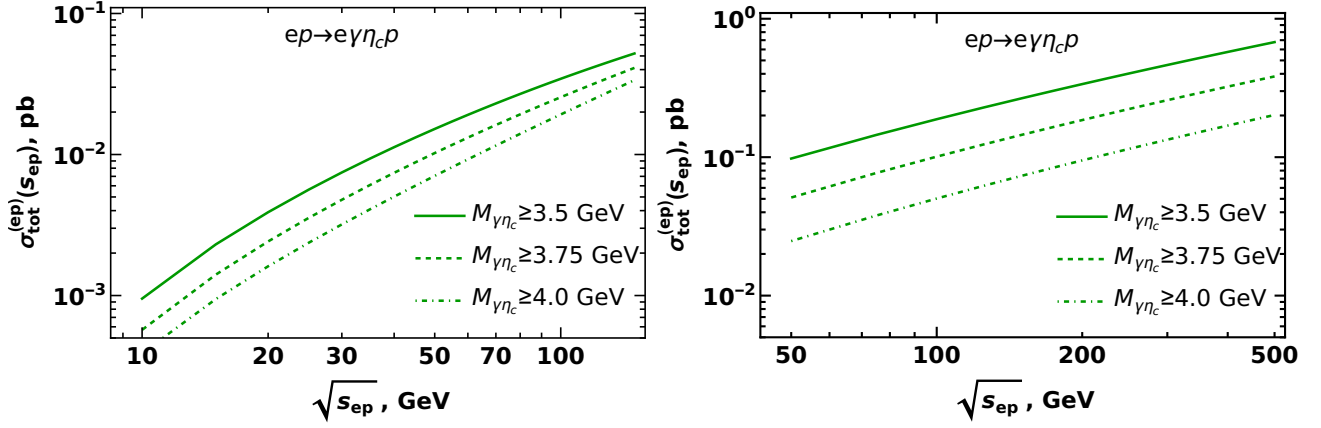
Figura 30: Predicciones para la sección eficaz total de la electroproducción de \gamma\eta_c en función de la energía \sqrt{s_{ep}} , para distintos cortes en la masa invariante de los pares \gamma\eta_c . El flujo de fotones se integró sobre la virtualidad hasta Q_{\text{max}}^2 \approx 1 \text{ GeV}^2 . Panel izquierdo: la factorización colineal; Panel derecho: el modelo del CGC.
