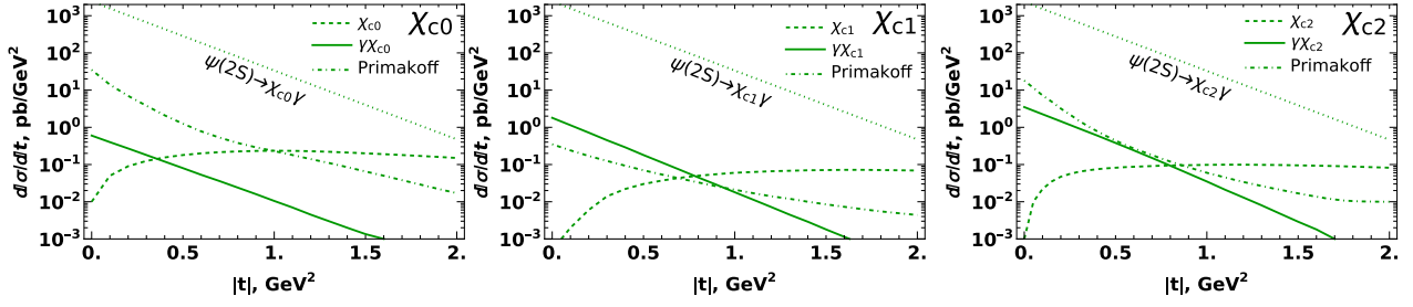
Figura 35: Comparación de la sección eficaz diferencial para distintos mecanismos que contribuyen a la fotoproducción exclusiva de \chi_{cJ} y de \gamma\chi_{cJ} (con el fotón final no detectado) a W = 35 \text{ GeV} (o x_{Bj} = 10^{-2} ). Las curvas sólidas corresponden al proceso directo \gamma p \rightarrow \gamma\chi_{cJ}p calculado en el marco de la factorización colineal. Las curvas punteadas superiores corresponden a la contribución de pares \gamma\chi_{cJ} procedentes de la desintegración radiativa \psi(2S) \rightarrow \gamma\chi_{cJ} . Las curvas para la fotoproducción exclusiva \gamma p \rightarrow \chi_{cJ}p mediada por odderón y el mecanismo de Primakoff se toman de [55].
