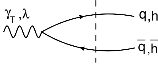
Figura 9: Diagrama correspondiente a la función de onda del fotón, con el vértice electromagnético y el denominador de energía del estado intermedio q\bar{q} (línea discontinua).
