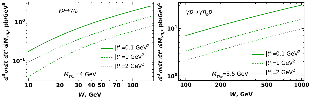
Figura 18: Dependencia de la sección eficaz diferencial en la energía W para \gamma\eta_c en la factorización colineal (panel izquierdo) y en el marco del CGC (panel derecho).
