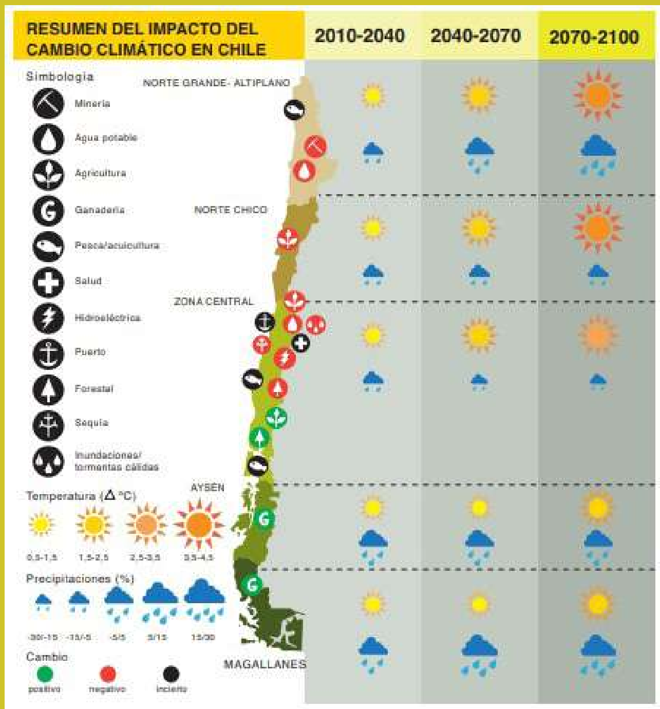
Fig. 67 Representación esquemática de los impactos del cambio climático y su relación con las proyecciones climáticas futuras. Fuente: CEPAL, 2012
