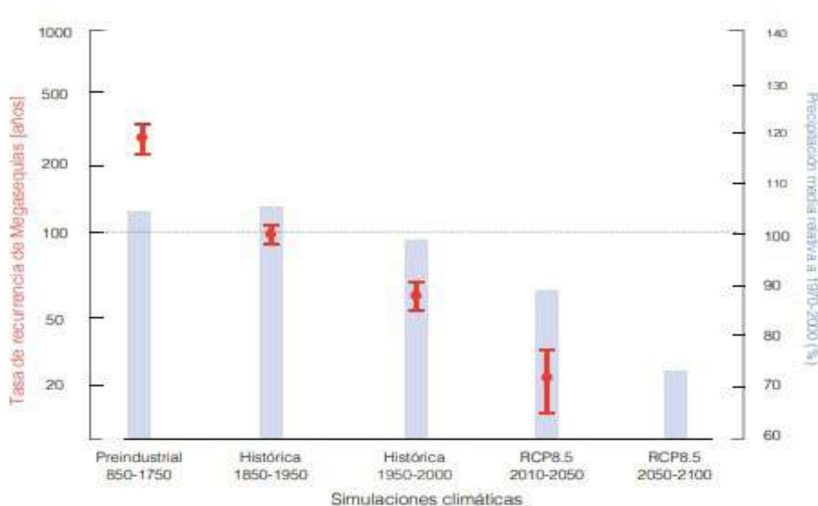
Fig. 78 Período de recurrencia en años (escala a la izquierda) de una sequía (>30% de déficit de precipitación en Chile central de tres o más años de duración, empleando siete modelos climáticos que simulan climas pasados, presentes y futuros. El período de recurrencia se calculó para cada modelo. Los círculos rojos indican el promedio y las líneas verticales la desviación estándar entre modelos. Las barras celestes indican el promedio multimodelo de la precipitación relativa a la media 1970-2000 (escala a la derecha). Datos: Coupled Model Intercomparison Project (CMIP5-WCRP). Fuente: CR2, 2015
