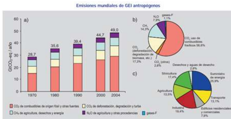
Figura RRP.3. a) Emisiones anuales mundiales de GEI antropógenos entre 1970 y 2004. a b) Parte proporcional que representan diferentes GEI antropógenos respecto de las emisiones totales en 2004, en términos de CO 2 equivalente. c) Parte proporcional que representan diferentes sectores en las emisiones totales de GEI antropógenos en 2004, en términos de CO 2 equivalente. (En el sector silvicultura se incluye la deforestación). (Figura 2.1)
