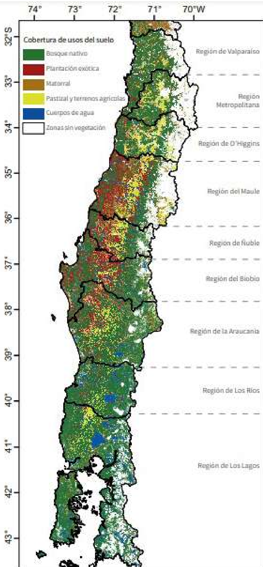
Fig. 88 Distribución geográfica de los diferentes usos de suelo entre las regiones de Valparaíso y Los Lagos. Fuente: Informe CR2 Incendios en Chile: Causas, impactos y resiliencia. (CR2, 2020)
