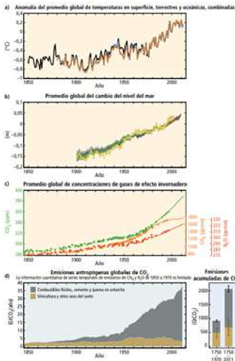
Figura 8B.1 | La compleja relación existente entre las observaciones (gráficos a, b y c, fondo amarillo-rosado) y las emisiones (gráfico d, fondo azul claro) se aborda en la sección 1.2 y en el tema 6. Observaciones y otros indicadores de un sistema climático global cambiante. Observaciones a) Anomalías del promedio anual y global de temperaturas en superficie, terrestres y oceánicas, combinadas respecto del promedio del período de 1950 a 2000. Los colores indican diferentes conjuntos de datos. b) Promedio anual y global del cambio del nivel del mar con respecto al promedio del conjunto de datos de más larga duración entre 1993 y 2000. Los colores indican diferentes conjuntos de datos. Todos los conjuntos de datos están alineados para tener el mismo valor en 1993, primer año de datos de altimetría por satélite (en rojo). En los casos en que se han evaluado los incrementos se indican mediante trazo de color. c) Concentraciones atmosféricas de los gases de efecto invernadero dióxido de carbono (CO 2 ), metano (CH 4 , naranja) y óxido nítrico (N 2 O, rojo) determinadas a partir de los datos de los testigos de hielo (verde) y de mediciones atmosféricas directas (rojo). Indicadores d) Emisiones antropogénicas globales de CO 2 , procedentes de la industria y otros usos del suelo y de la quema de combustibles fósiles, la producción de cemento y la quema en agricultura. Las emisiones acumuladas de CO 2 de esas fuentes y sus incertidumbres se muestran como barras y líneas azules, respectivamente, a la derecha. Los efectos globales de la acumulación de emisiones de CO 2 y N 2 O se muestran en el gráfico c. Los datos de las emisiones de gases de efecto invernadero de 1970 a 2010 se muestran en la Figura 8B.2. (Figuras 1.1, 1.3, 1.5)
