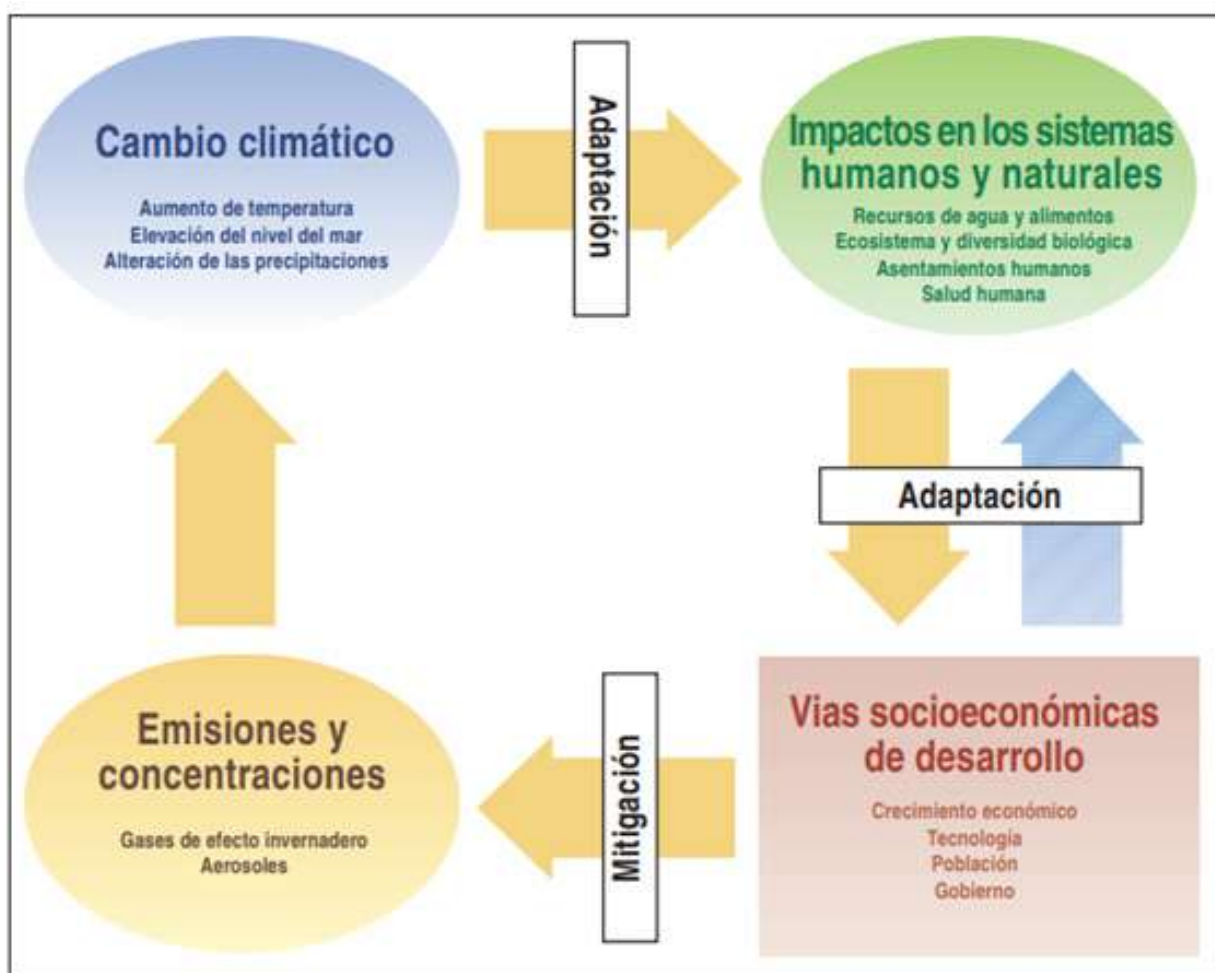
Figura RRP-1: Cambio climático—un marco integrado. Representación esquemática y simplificada de un marco de evaluación integrado para la consideración de los cambios climáticos antropogénicos. Las flechas amarillas muestran el ciclo de causa a efecto entre los cuatro cuadrantes mostrados en la figura, y la flecha azul indica la respuesta de la sociedad ante los impactos del cambio climático. Véase una descripción más detallada de este marco, al pie de la Figura 1-1.
