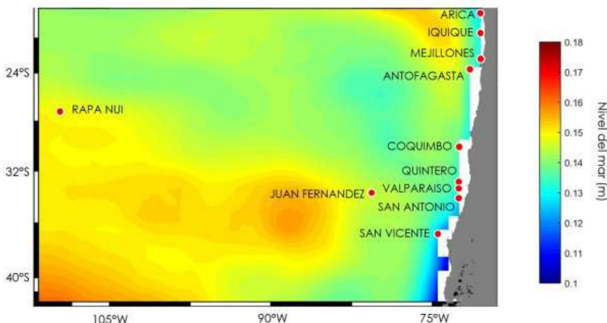
Fig. 73 Incremento del nivel del mar respecto entre la mediana de la proyección (2026-2045) respecto de la mediana del período histórico (1986-2005). Los puntos rojos corresponden a los nodos más cercanos a los puertos en los cuales se efectúa la proyección. Ministerio del Medio Ambiente, 2019. Volumen 1: Amenazas en “Determinación del riesgo de los impactos del cambio climático en las costas de Chile” Fuente: MMA, 2019
