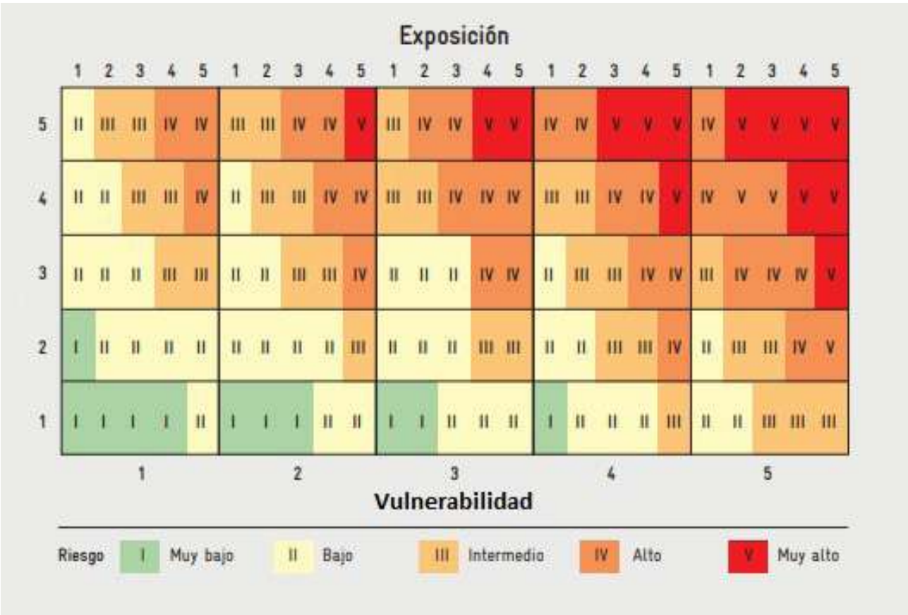
Fig. 97 Matriz para el cálculo de riesgo con las tres variables asociadas (amenaza, exposición y vulnerabilidad). Fuente: Libro de la Vulnerabilidad. (GIZ & EURAC, 2014).
