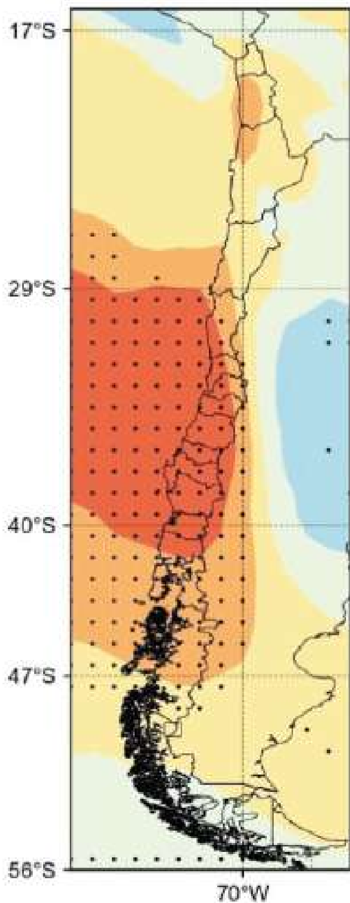
SSP370
