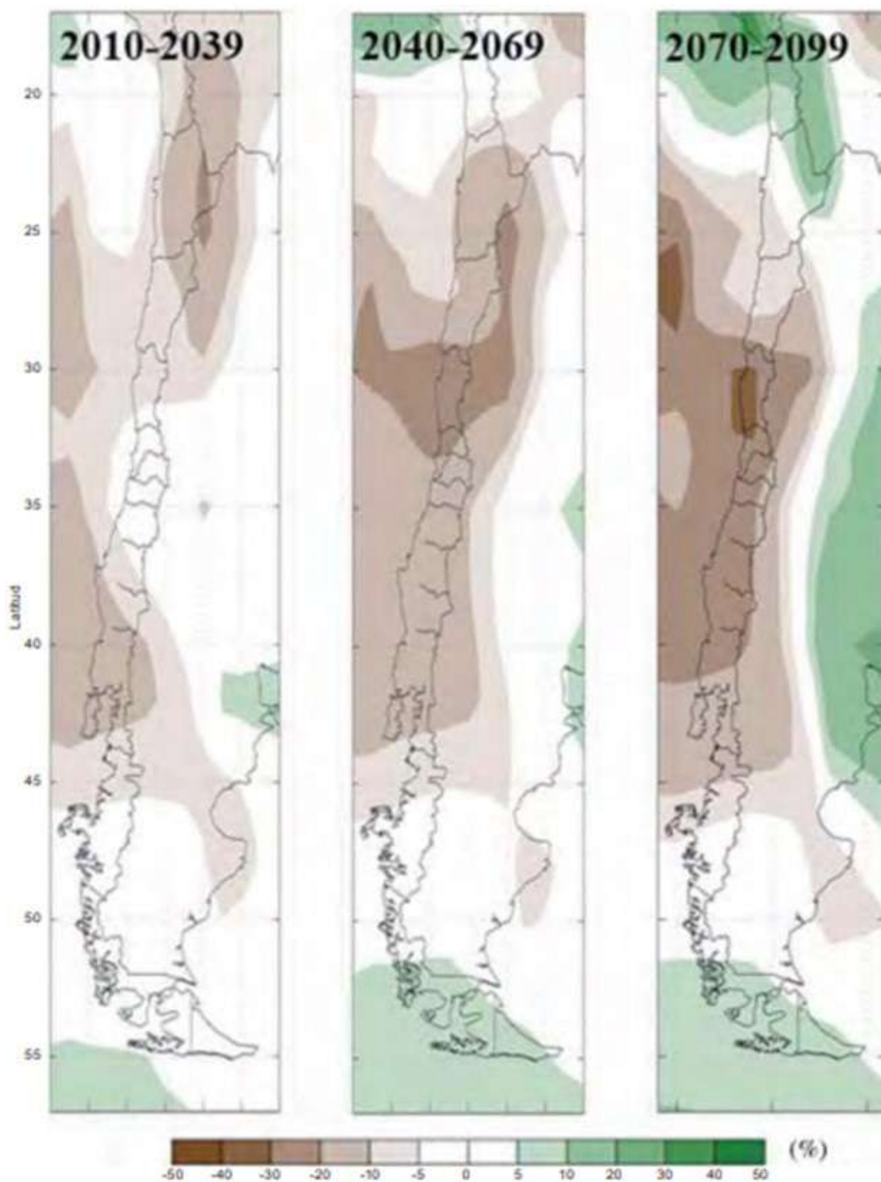
Fig. 54 Mapa de Chile en donde se grafica la proyección de precipitaciones en base al escenario A2 en 3 periodos de tiempo, 2010 al 2039, del 2040 al 2069, y del 2070 al 2099. Fuente: CEPAL, 2012
