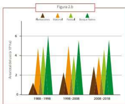
Figura 2.b. Área total de cada uso del suelo (entre Valparaíso y Los Lagos). Datos extraídos de Heilmayr et al. (2016).
