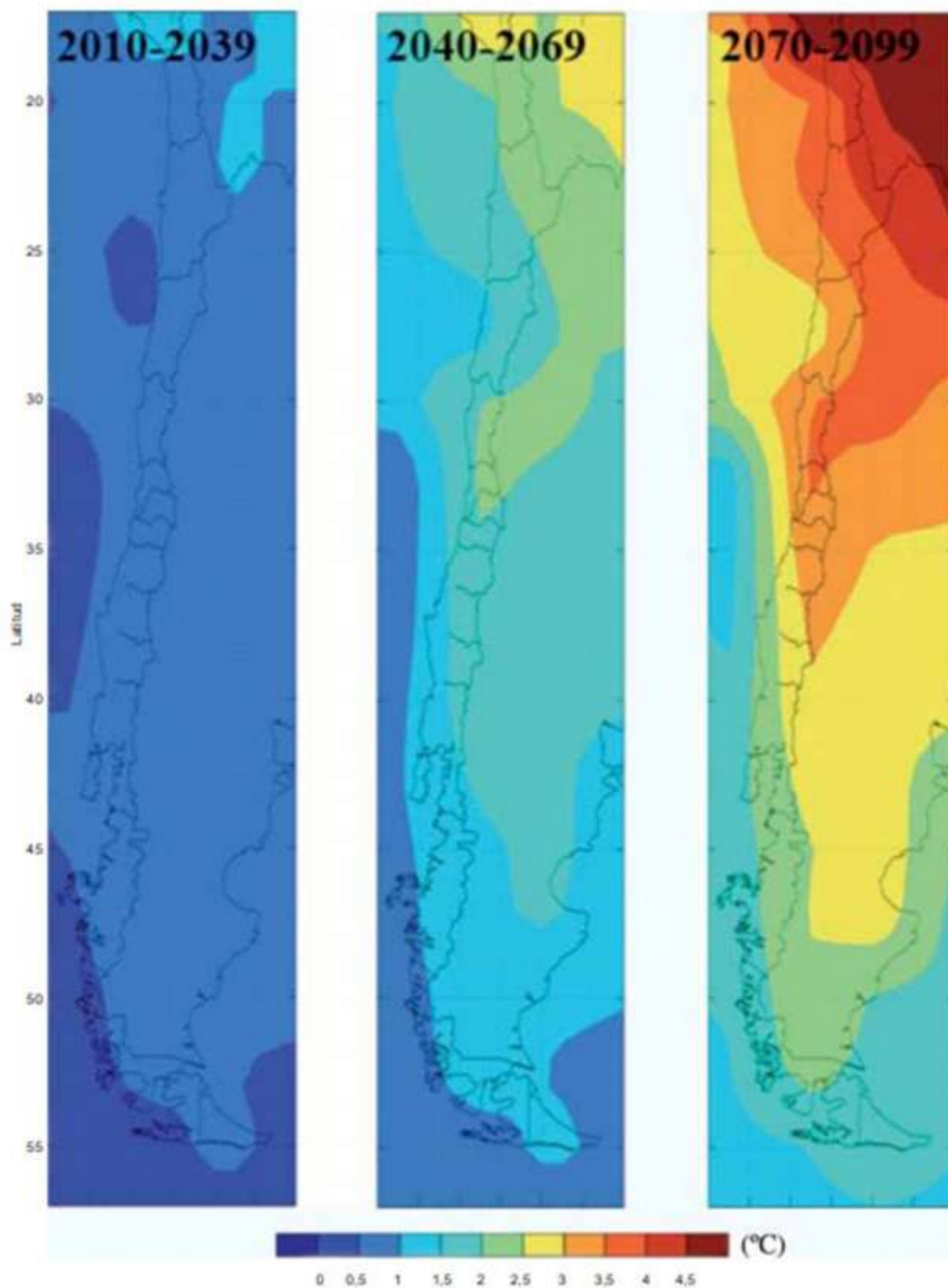
Fig. 52 Mapa de Chile en donde se grafica la proyección de temperatura en base al escenario A2 en 3 periodos de tiempo, 2010 al 2039, del 2040 al 2069, y del 2070 al 2099. Fuente: CEPAL, 2012
