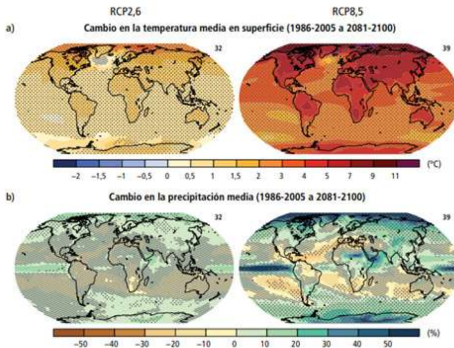
Figura RRP.7 | Cambio en la temperatura media en superficie (a) y cambio en la precipitación media (b) sobre la base de las proyecciones de la media multimodelos para 2081-2100 en relación con 1986-2005 bajo los escenarios RCP2.6 (izquierda) y RCP8.5 (derecha). En la esquina superior derecha de cada mapa se indica el número de modelos utilizados para calcular la media multimodelos. Las tramas punteadas indican las regiones donde el cambio proyectado es grande con respecto a la variabilidad interna natural y donde al menos el 90% de los modelos concuerdan con el signo del cambio. Las tramas rayadas (líneas diagonales) muestran las regiones donde el cambio proyectado es inferior a una desviación típica de la variabilidad interna natural. (2.2, figura 2.2)
