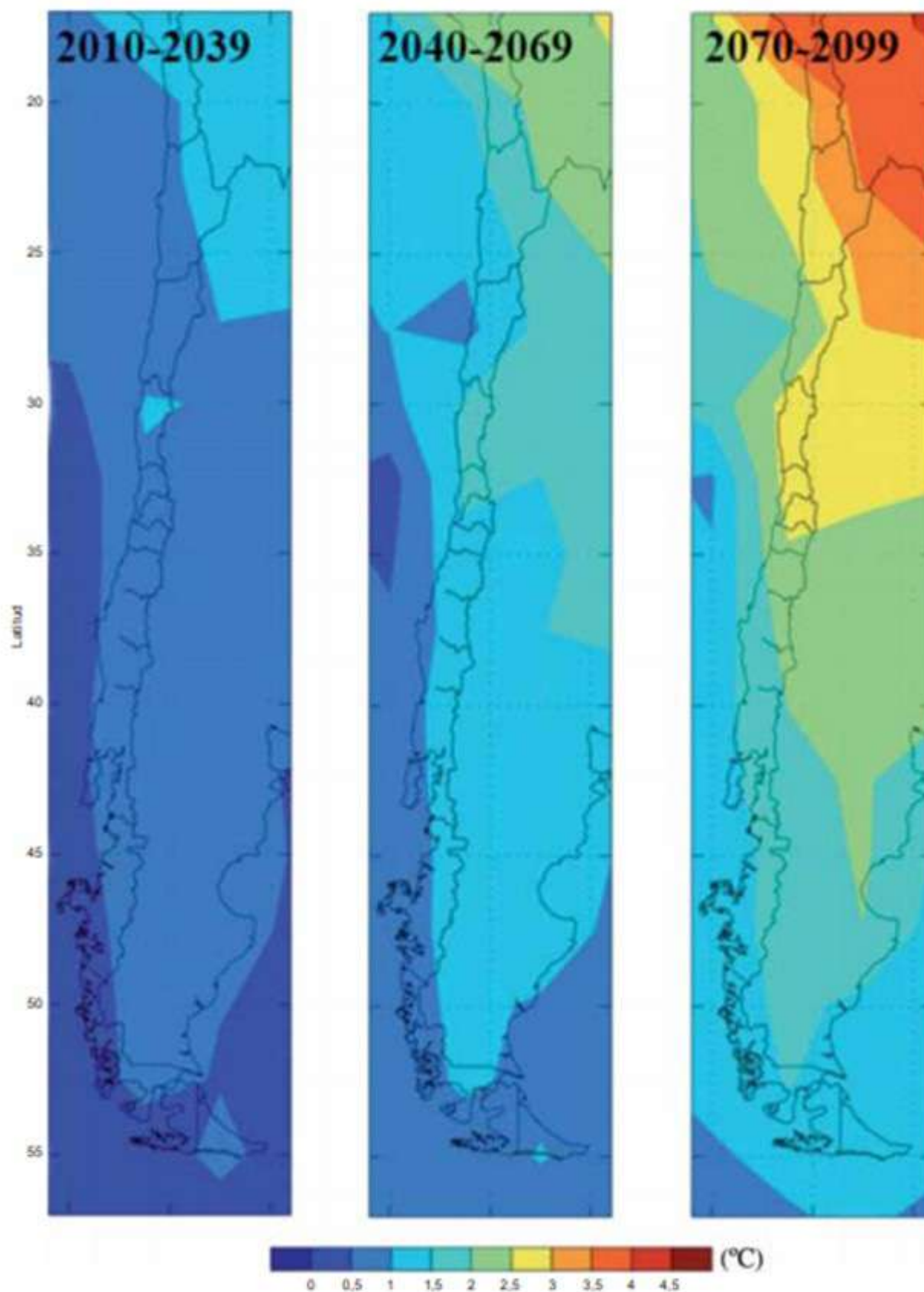
Fig. 53 Mapa de Chile en donde se grafica la proyección de temperatura en base al escenario B2 en 3 periodos de tiempo, 2010 al 2039, del 2040 al 2069, y del 2070 al 2099.
