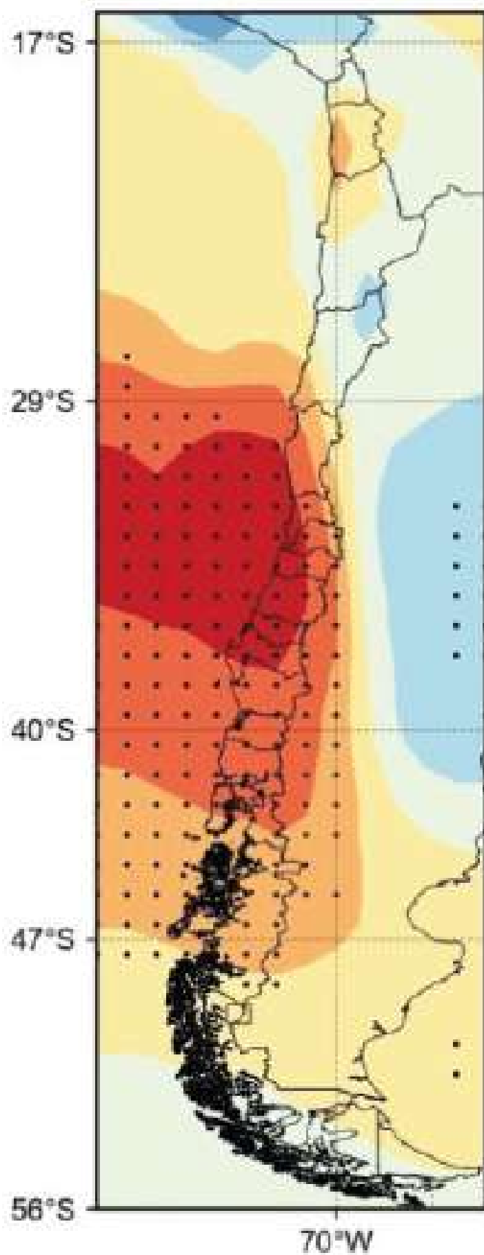
SSP585
