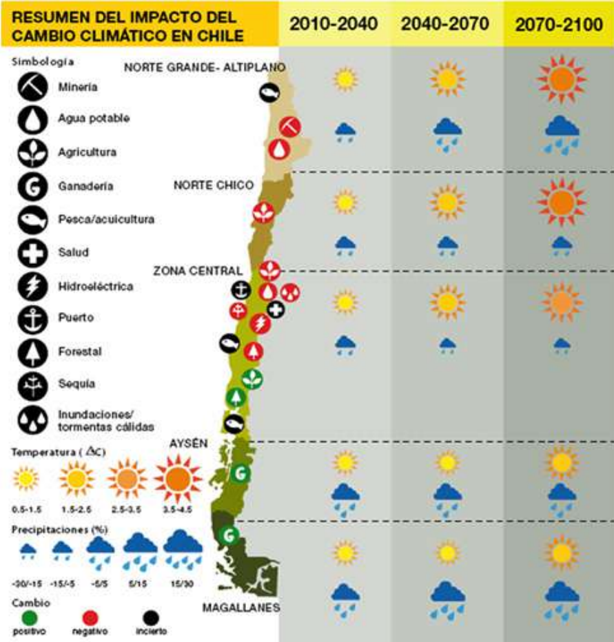
Fig. 6 Resumen del impacto del cambio climático en las actividades económicas en Chile, en el periodo del 2010-2100. Fuente: CEPAL, 2012
