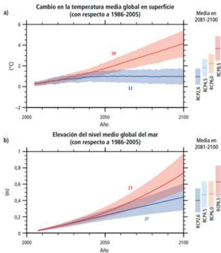
Figura RRP.6 | Cambio en la temperatura media global en superficie (a) y elevación del nivel medio global del mar (b) de 2006 a 2100 determinados por simulaciones multimodelos. Todos los cambios son en relación con 1986-2005. Las series temporales de las proyecciones y la medición de la incertidumbre (sombreado) se muestran en relación con los escenarios RCP2.6 (azul) y RCP8.5 (rojo). Las incertidumbres medias y asociadas, promediadas entre 2081 y 2100, figuran en todos los escenarios de RCP indicadas con barras verticales de colores en el margen derecho de cada gráfico. Se indica asimismo el número de modelos de la quinta fase del Proyecto de comparación de modelos acoplados (CMIP5) utilizados para calcular la media multimodelos. (2.2, figura 2.1)
