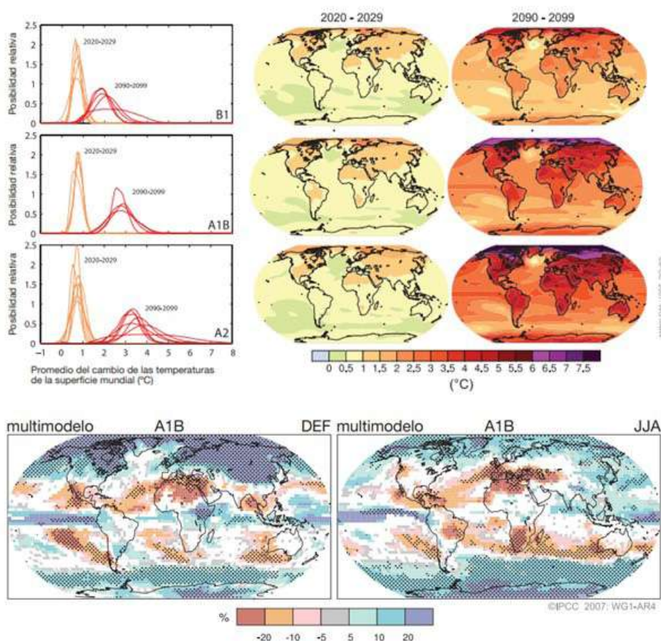
Fig. 50 Proyecciones de las temperaturas de la superficie para principios y finales del siglo XXI con respecto al periodo 1980–1999. Los paneles centrales y el derecho muestran el promedio de las proyecciones multi-modelos MCGAO para los escenarios IE-EE I B1 (arriba), A1B (en el medio) y A2 (abajo) promediados en las décadas 2020–2029 (centro) y 2090–2099 (derecha). Los paneles a la izquierda muestran las incertidumbres correspondientes como probabilidades relativas del calentamiento medio mundial estimado en varios estudios de MCGAOs y del Modelo del Sistema Terrestre de Complejidad Intermedia para los mismos periodos. Algunos estudios solo presentan los resultados de un subconjunto de escenarios del IE-EE, o de varias versiones de los modelos. Por tanto, la diferencia en el número de curvas mostradas en los paneles de la izquierda sólo se debe a diferencias en la disponibilidad de los resultados. Fuente: IPCC, 2007
