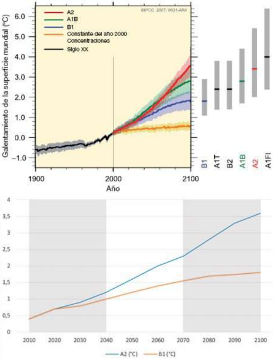
Fig. 49 Gráfico donde se comparan los aumentos de temperatura de los escenarios A2 y B1. La línea azul representa el escenario A2, mientras que la línea naranja representa el escenario B1. Fuente: Reelaboración basada en el IPCC de 2007.
