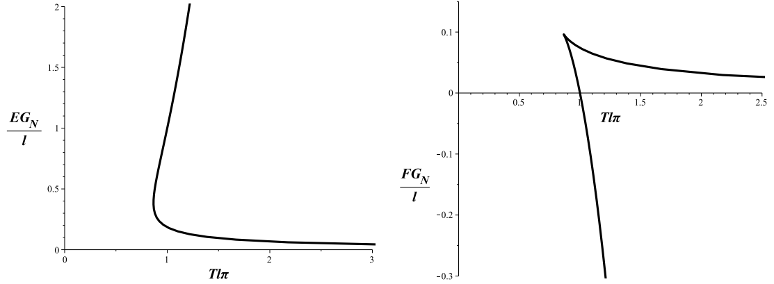
Figura 4.1: Ambas figuras son para los agujeros negros de Schwarzschild-AdS. Izquierda, E vs T y Derecha F vs T. En la figura G_N es la constante de Newton, pero a lo largo de la tesis usaremos G .
