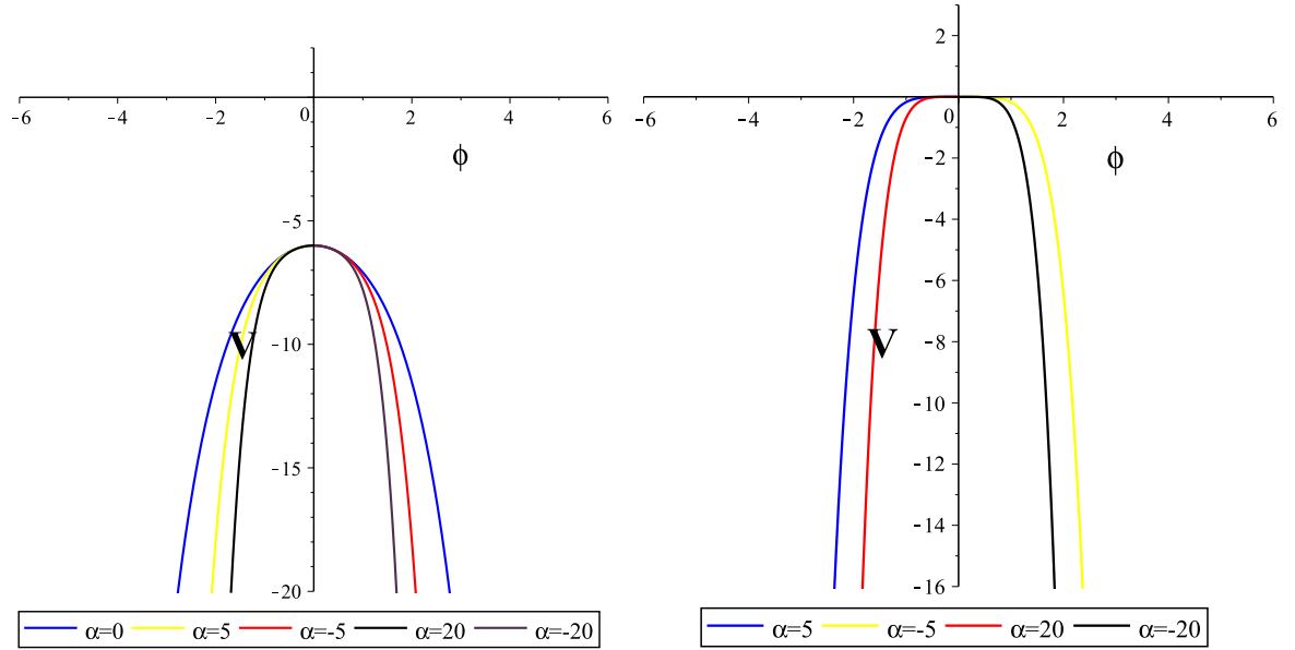
Figura 3.1: En nuestra notación: V = V(\phi) , \phi(x) = \ln x . La figura de la izquierda es el potencial para teorías asintóticamente AdS. La figura de la derecha es el potencial para teorías asintóticamente planas.
