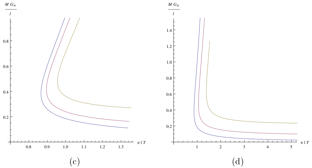
Figura 6.2: (c) Masa adimensional versus temperatura adimensional, para diferentes valores de \nu , \alpha = 10l^{-2} y campo escalar negativo. Los graficos son para \nu = 1 , \nu = 1,9 y \nu = 3 (de izquierda a derecha). Aquí es posible ver la existencia de pequeños y grandes agujeros negros, exáctamente similar a Schwarzschild AdS.
