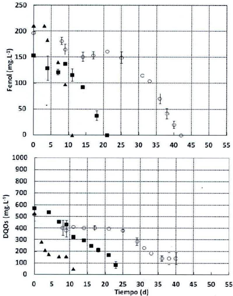
Figura 5.13: Concentración de fenol y DQOs en ensayo de adiciones sucesivas de 200 \text{ mg}\cdot\text{L}^{-1} de fenol, utilizando un inóculo de una planta de tratamiento de una industria de tabaco.
