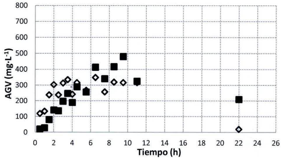
Figura 4.5: Concentración de AGVs operando en estado estacionario a 37°C (Ácido acético (◇), ácido propiónico (■)).
