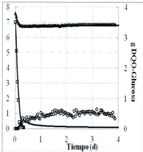
Figura 4.15: Ajuste de datos de producción de biogás (O), glucosa (□) y pH (Δ) a 37°C (A), 31°C (B), 25°C (C) y 20°C (D).
