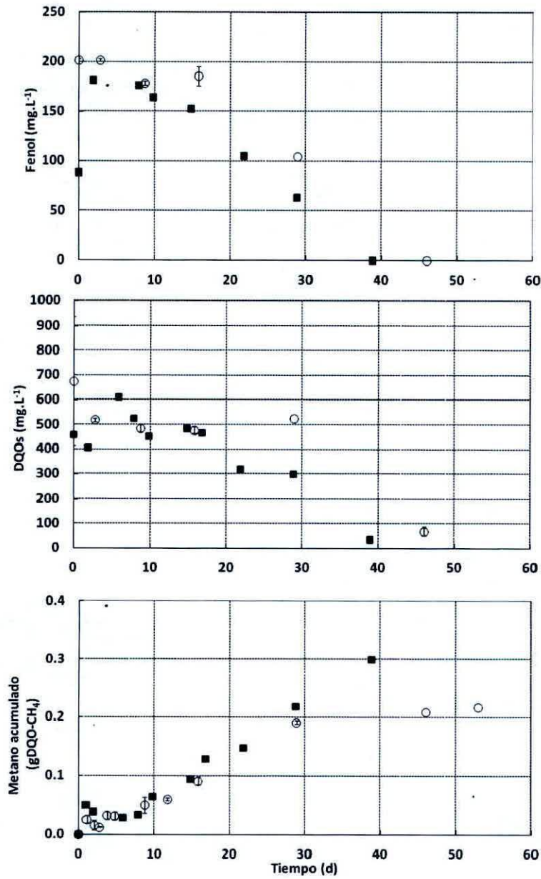
Figura 5.12: Metano acumulado, concentración de fenol y DQOs en ensayo de adiciones sucesivas de 200 mg·L -1 de fenol. Inóculo planta de tratamiento de cerveza.
