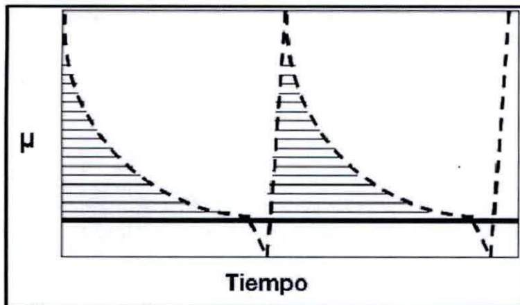
Figura 2.3: Comparación de la productividad de un sistema continuo y uno por lotes secuenciales. Lotés (---) continuo (—). La zona achurada representa la ganancia de productividad de un sistema por lotes por sobre un continuo (Donoso-Bravo, 2008).
