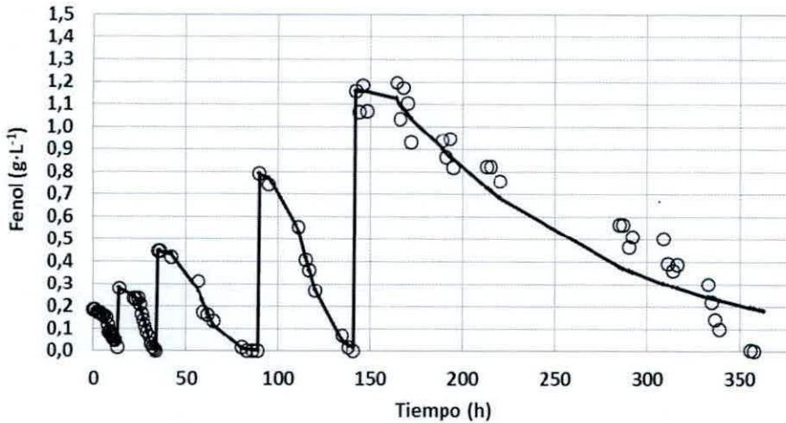
Figura 5.19: Ajuste de datos de degradación anaerobia de fenol. Simulación (—); datos experimentales (○), a 120, 240 500, 800 y 1200 \text{mg}\cdot\text{L}^{-1} de fenol.
