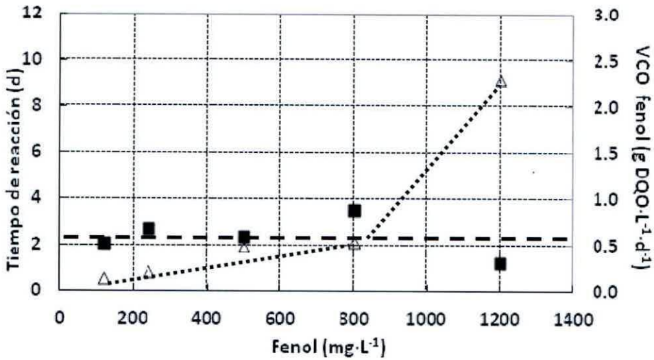
Figura 5.16: VCO (■) y tiempo de reacción (Δ) en el último ciclo de operación a diferentes concentraciones de fenol ( 120, 240, 500, 800 and 1200 \text{ mg phenol}\cdot\text{L}^{-1} ) en reactor ASBR. La línea punteada representa la VCO promedio.
