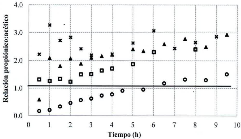
Figura 4.9: Relación concentración propiónico: acético operando en estado estacionario a diferentes temperaturas (37°C (O), 31°C (□), 25°C (▲), y 20°C (×)). La línea indica el valor límite de 1.
