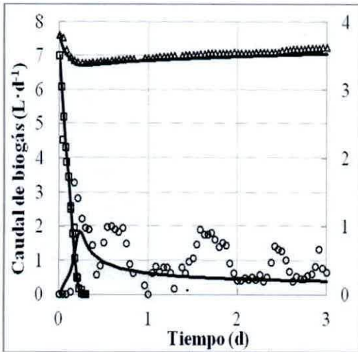
Figura 4.15: Ajuste de datos de producción de biogás (O), glucosa (□) y pH (Δ) a 37°C (A), 31°C (B), 25°C (C) y 20°C (D).
