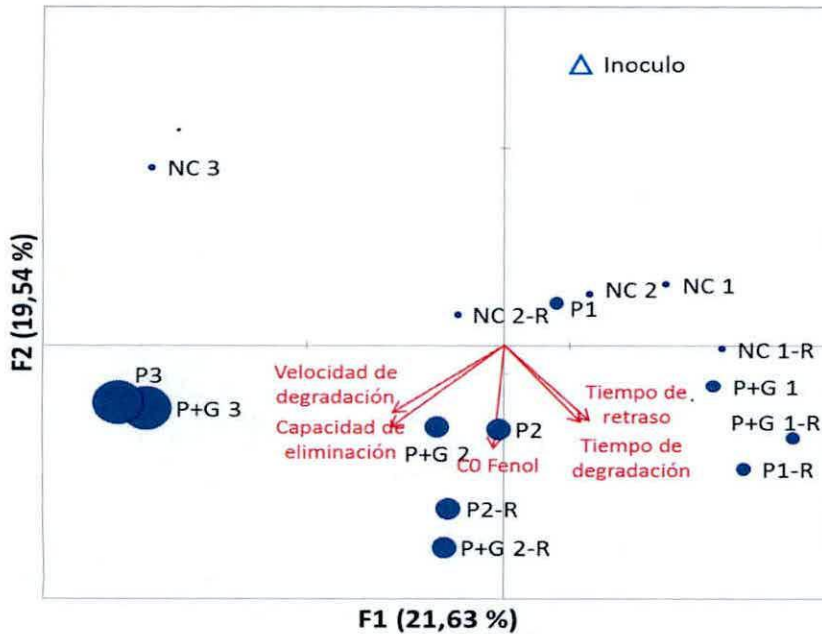
Figura 6.2: Análisis de Componentes Principales (PCA) de perfiles de DGGE de ensayos en batch (botellas). El tamaño del símbolo es proporcional a la velocidad de degradación de fenol. El sustrato es indicado por P (solo Fenol) o P+G (Fenol+Glucosa). 1-2-3: número de adiciones de fenol. R: replica de ensayos; NC: control negativo.
