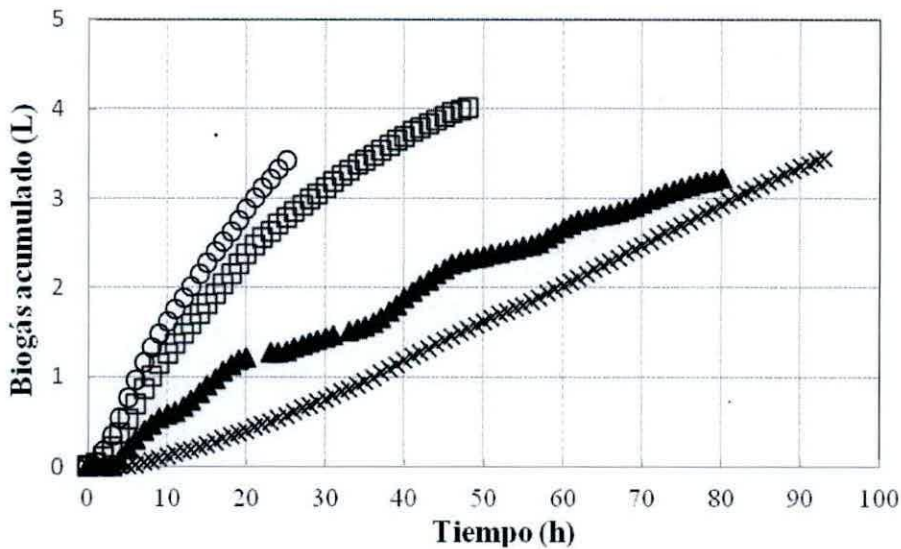
Figura 4.12: Biogás acumulado a las diferentes temperaturas (37°C (O), 31°C (□), 25°C (▲), 20°C (×)).
