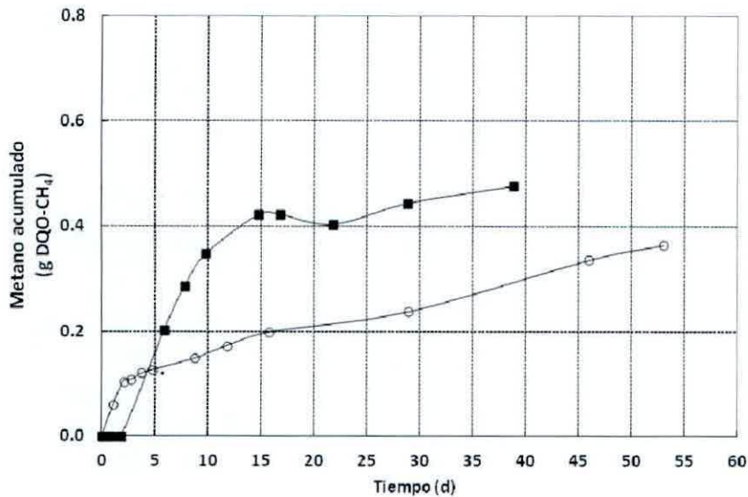
Figura 5.8: Metano acumulado en ensayos sin adición de sustrato (blanco) de degradación anaerobia de fenol utilizando biomasa de planta de tratamiento de una industria cervecera. Blanco de ensayo de primera adición de fenol (■); segunda adición de fenol (○).
