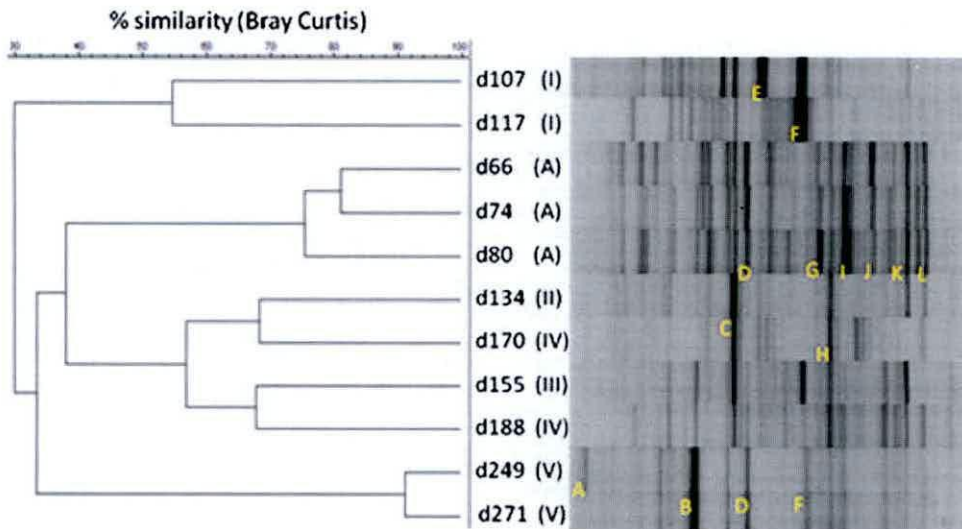
Figura 6.3: Dendrograma UPGMA de los perfiles de DGGE de las muestras del reactor ASBR basado en el análisis de similaridad Bray Curtis. El número indica la concentración de entrada de fenol (medida) al comienzo de cada ciclo de operación.
