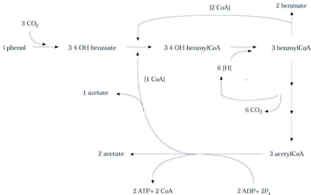
Figura 5.2: Propuesta de vía de degradación de fenol, basado en resultados preliminares de transformación de fenol a benzoato y acetato en botellas-modificadas con BES. El fenol es inicialmente reducido, formando benzoyl CoA, desde 4-Hidroxybenzoil-CoA. En la etapa de reducción son consumidos 6 [H]. Un tercio de 4 hidroxybenzoyl CoA es oxidado a acetato durante la formación de 6 [H]. El 4-Hidroxybenzoil-CoA remanente es convertido a benzoato (Karlsson et al. , 1999).
